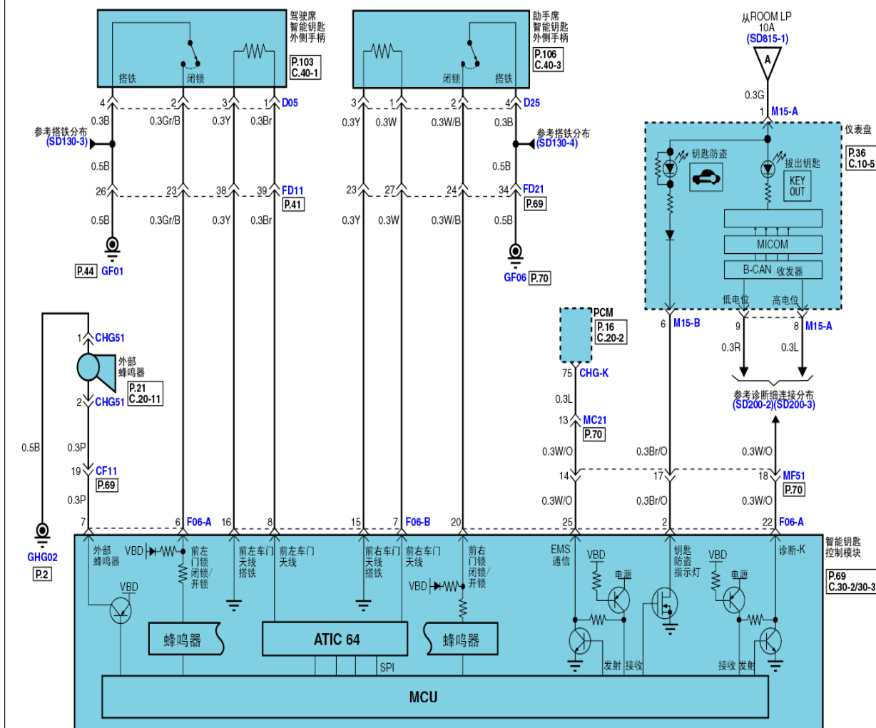
智能钥匙系统 (2)
