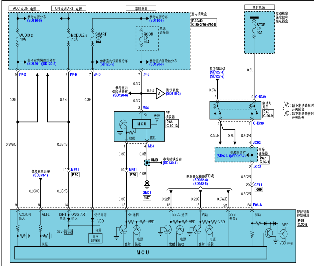
智能钥匙系统 (1)
