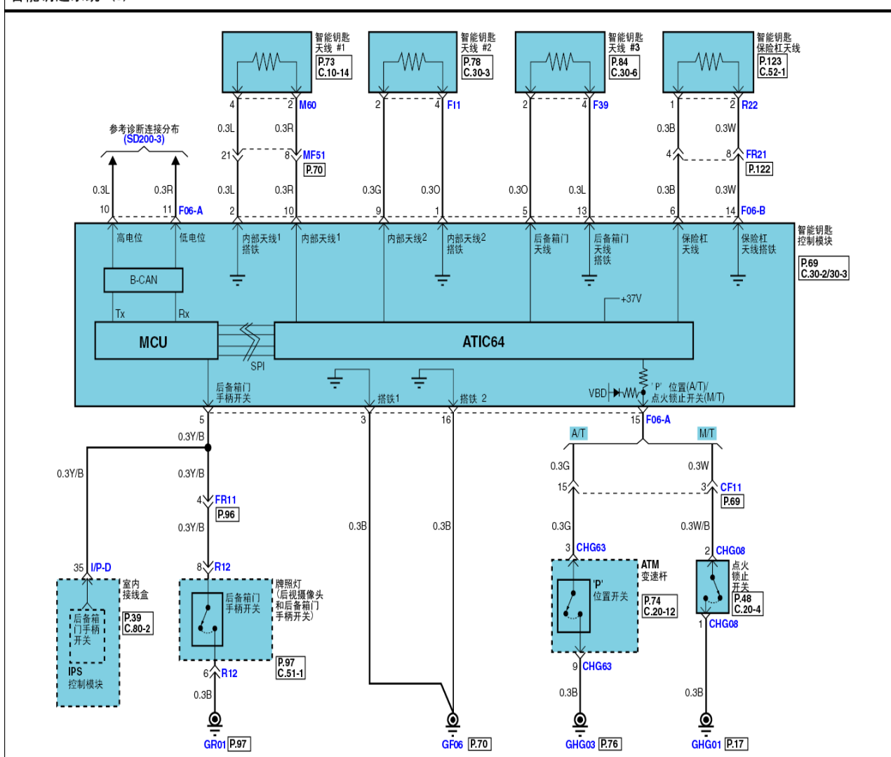
智能钥匙系统 (3)
